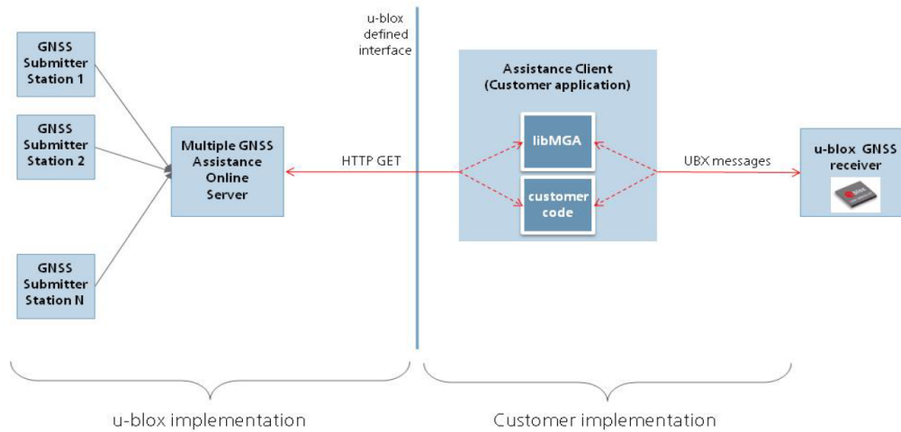
Figure 26: MGA architecture
