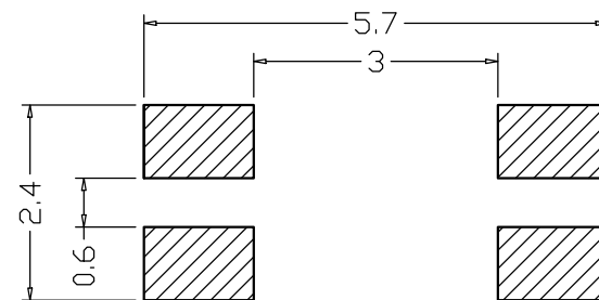
PCB线路板图
